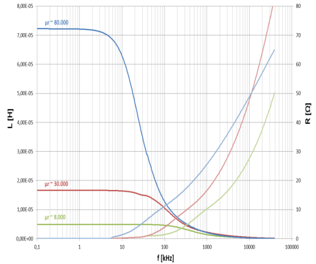
Induktivität und Serienwiderstand / Inductivity and Series Resistance (Kerngröße / core size 63 x 50 x 30mm)
