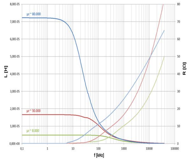
Induktivität und Serienwiderstand / Inductivity and Series Resistance (Kerngröße / core size 63 x 50 x 30mm)
