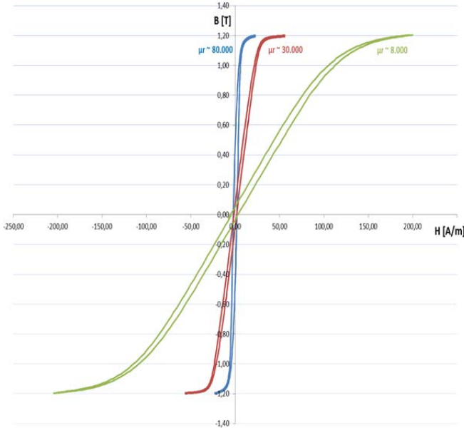
Hystereseschleifen (quasistatisch, 50 Hz) / Hysteresis loop (quasistatic, 50 Hz)
