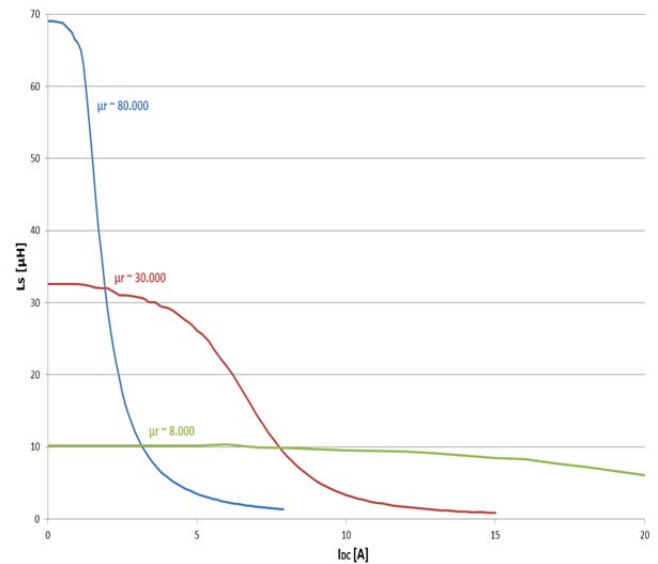
Vormagnetisierung / DC behaviour (Kerngröße / core size 63 x 50 x 30mm)
