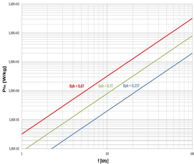
Verluste (Bpk = Induktions-Spitzenwert, sin) / Losses (Bpk = Induction peak, sin)
