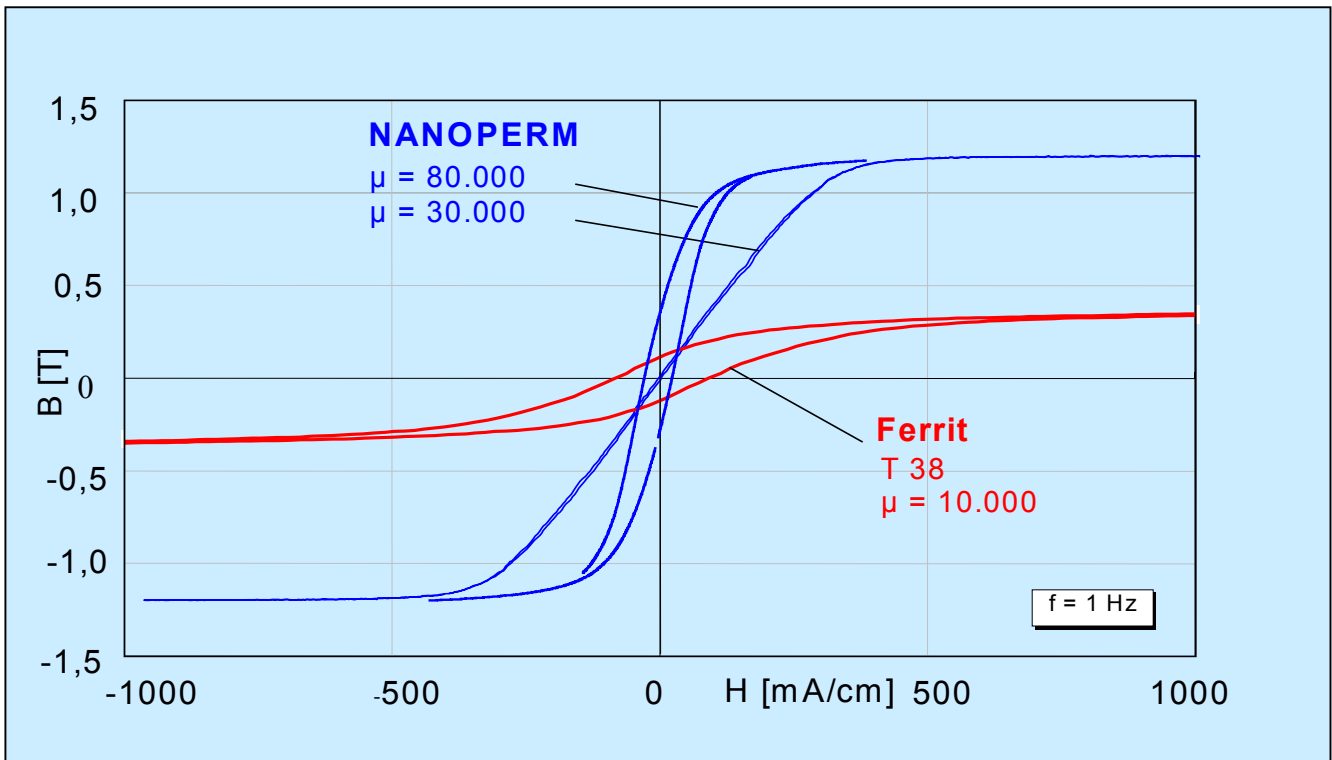
Hysteresen, Sättigungsfeldstärke bei variabler Permeabilität
