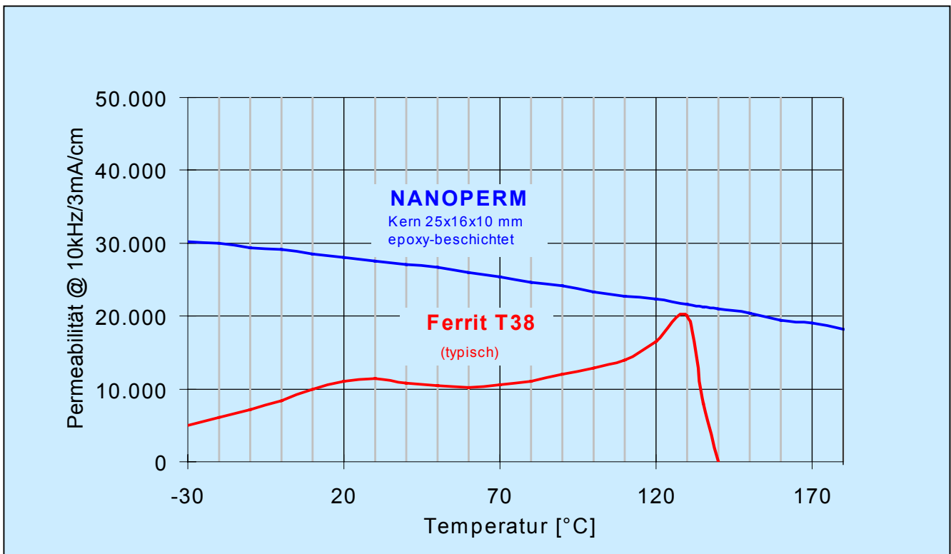
Permeabilität über die Temperatur
